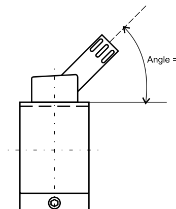
Typ E sonderausführung, Angabe: Winkel und Richtung / Type, custom design, Specife: angle and direction
