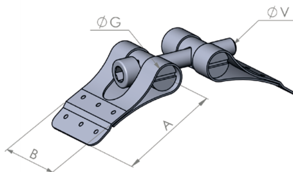
Abbildung: KLEMME-ZUSAMMENSETZUNG / Drawing: CLAMP ASSEMBLY
