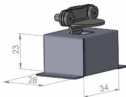
CV-10 RADIAL Anschlussbox / Connection box
